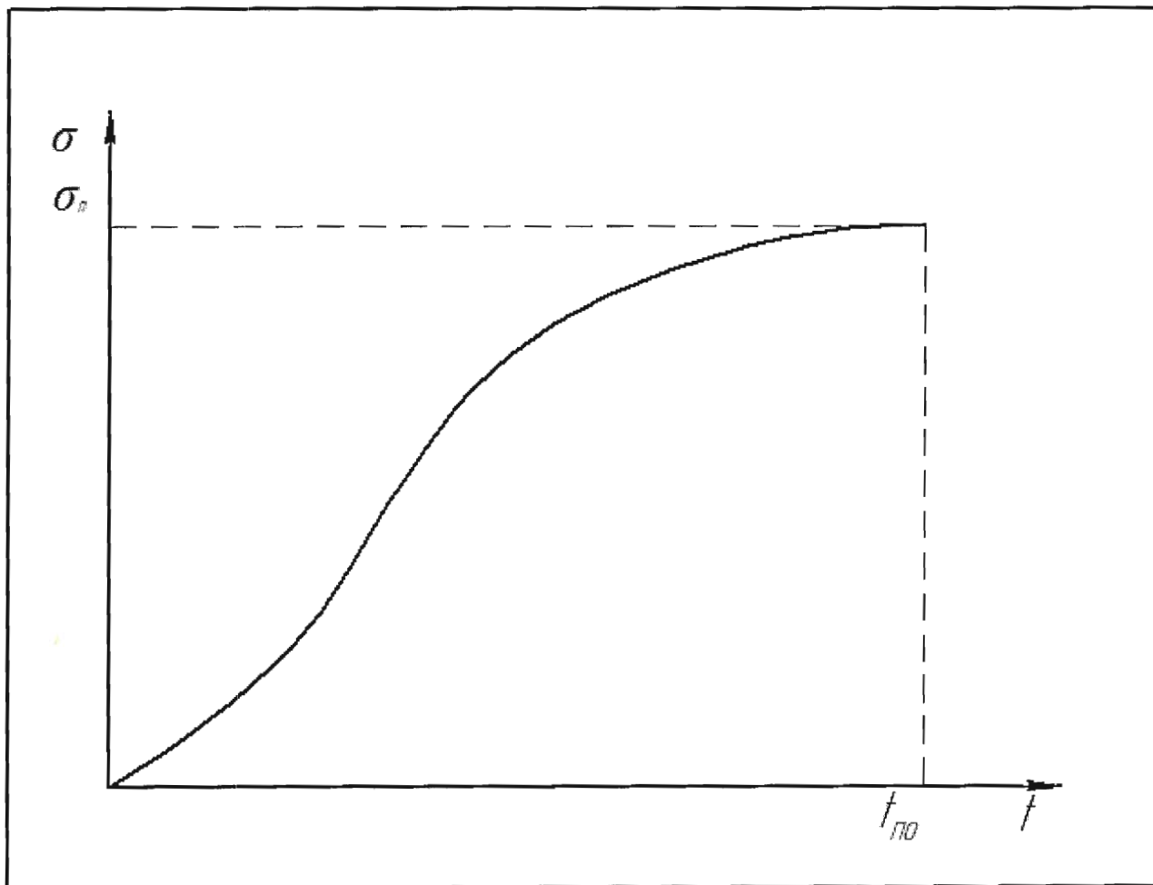
Рисунок Б.1 – Зависимость прочности клеевого образца \sigma от времени отверждения t
